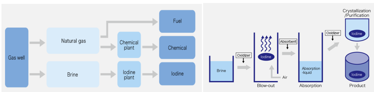
Figura 9: Schema del processo di produzione dello iodio dai pozzi di estrazione del gas naturale in Giappone
